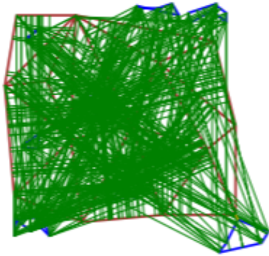
Abbildung 3: Visualisierung: hund03.txt
