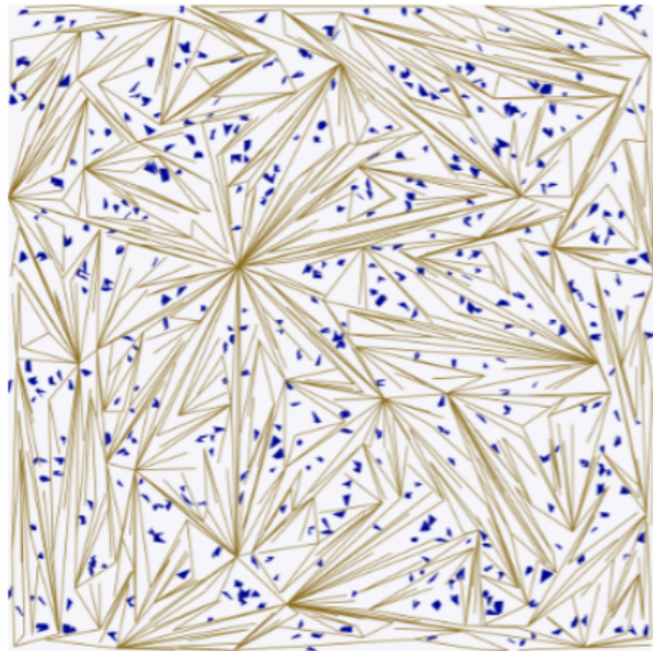
Abbildung 3: Visualisierung: hund03.txt
