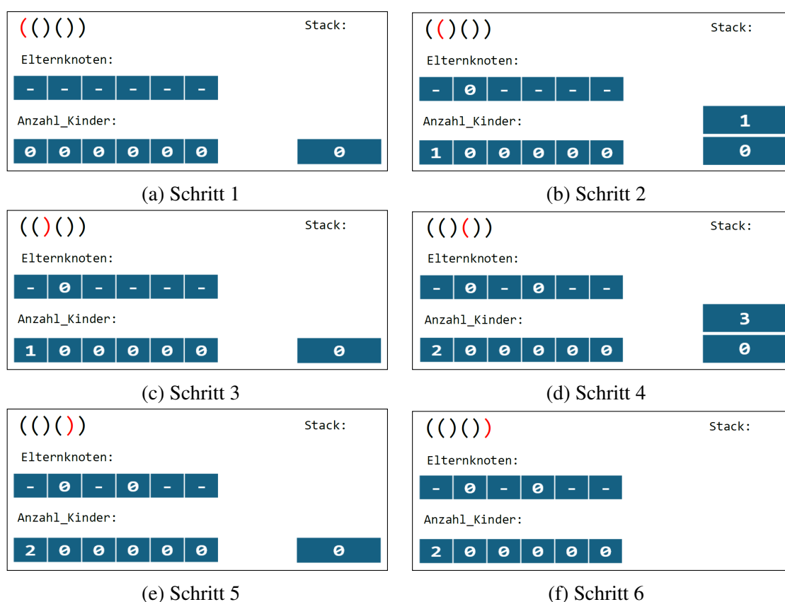
Abbildung 1.1: Die Abbildungen (a) bis (f) stellen das Vorgehen bei der schrittweisen Verarbeitung der Eingabe ((()())) dar. Es ist jeweils zu sehen, welche Eingabe gelesen wird, wie sich das Array der Elternknoten und Kindknoten verändert und welche Werte auf dem Stack liegen.
