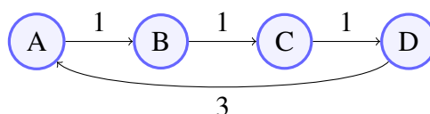
Abbildung 2.1: Distanzberechnung
